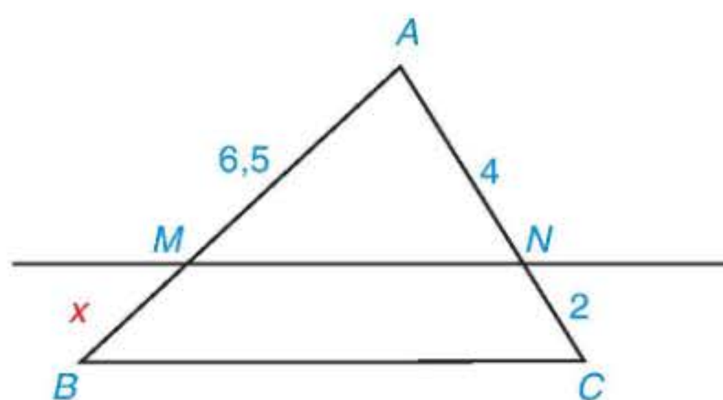
a) MN \parallel BC
